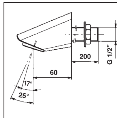
Dosah sprchy při úhlu 25° (E)
