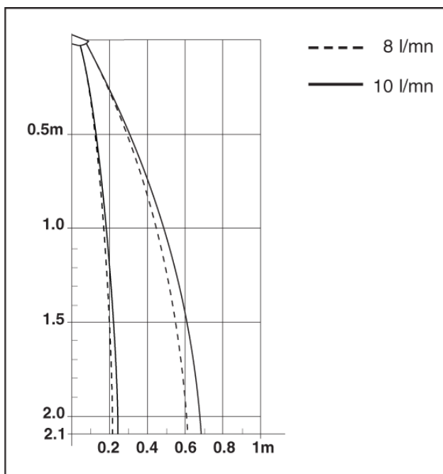
Dosah sprchy při úhlu 17° (D)
