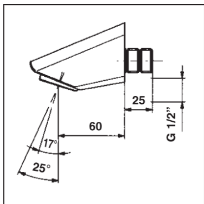
Dosah sprchy při úhlu 17° (D)
