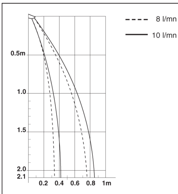
Dosah sprchy při úhlu 25° (E)
